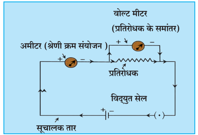
3.5 विद्युत परिपथ
