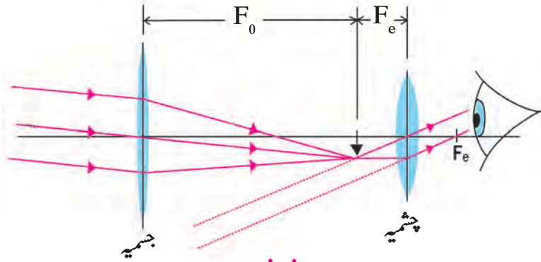
7.18: آخری دوربین
