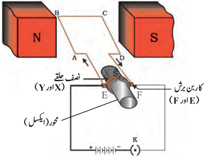
4.13: برقی موٹر - اصول اور کارکردگی
