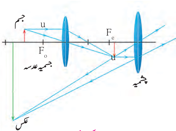
7.17: مرکب خوردبین
