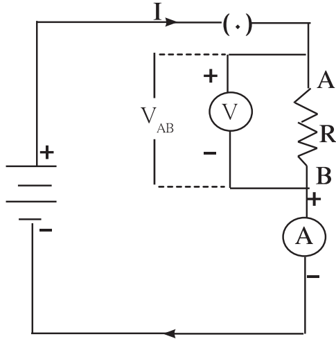
4.2: برقی رو
