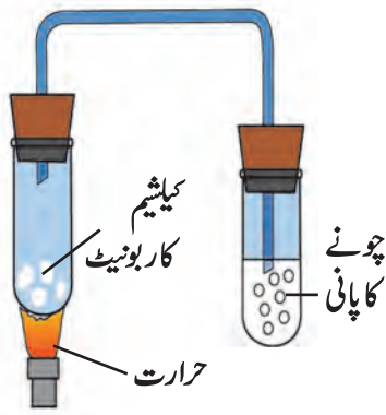
3.6: کیمیائے کاربونیٹ کا تجزیہ
