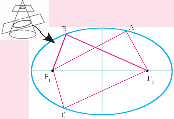
1.3: بیضوی مدار
