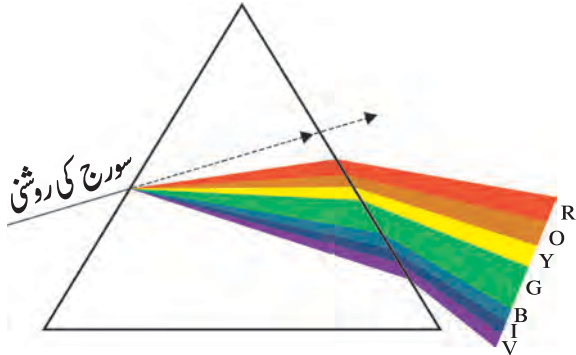
6.8: نور کا بکھرنا
